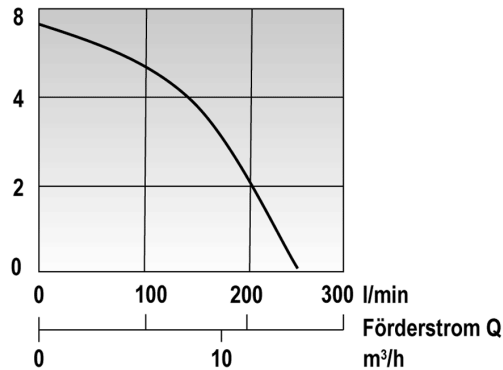
Förderhöhe H m (WS)
