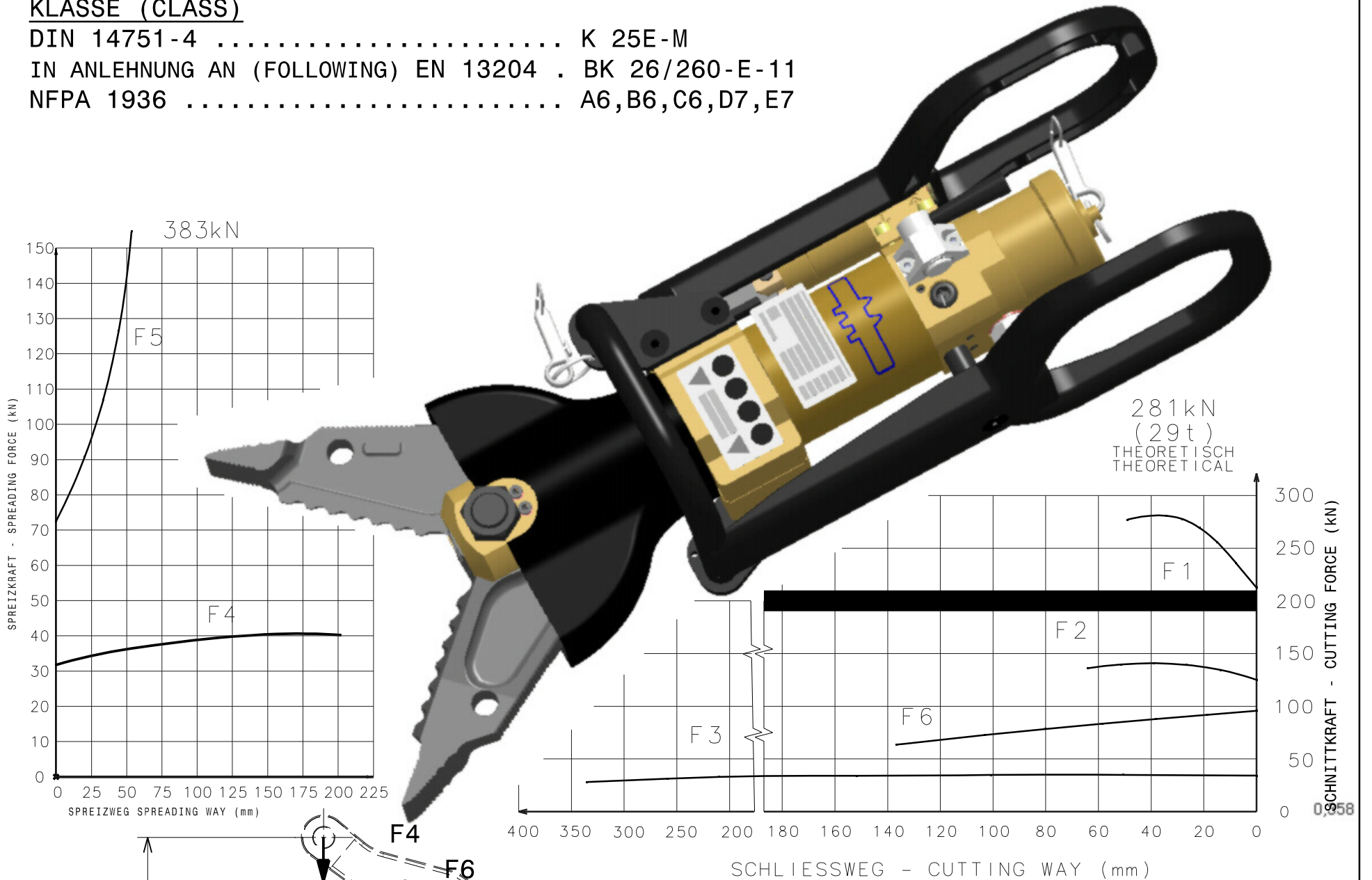
ALLE KRÄFTE BEI 63 MPa U. OHNE WIRKUNGSGRAD DIAGRAMM AT 63 MPa AND WITHOUT EFFICIENCY
